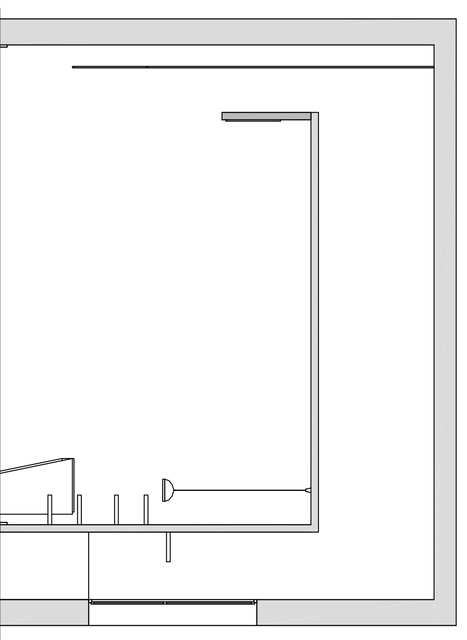
Sezione C-C'
