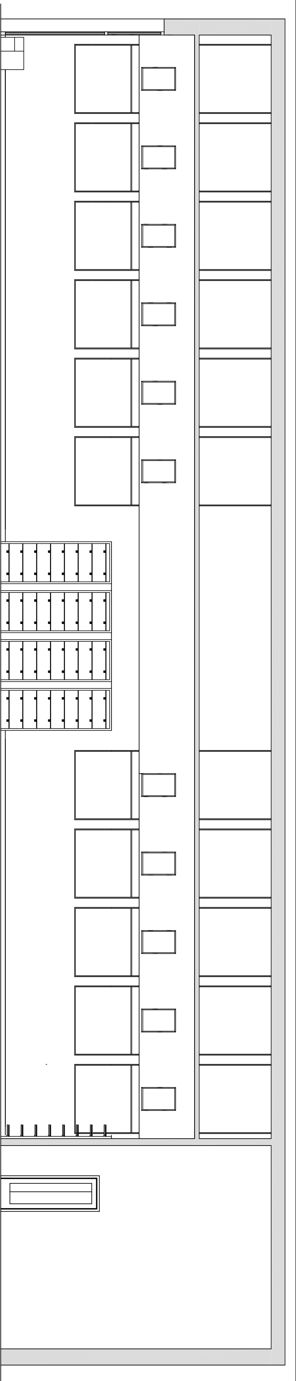
Sezione A-A'
